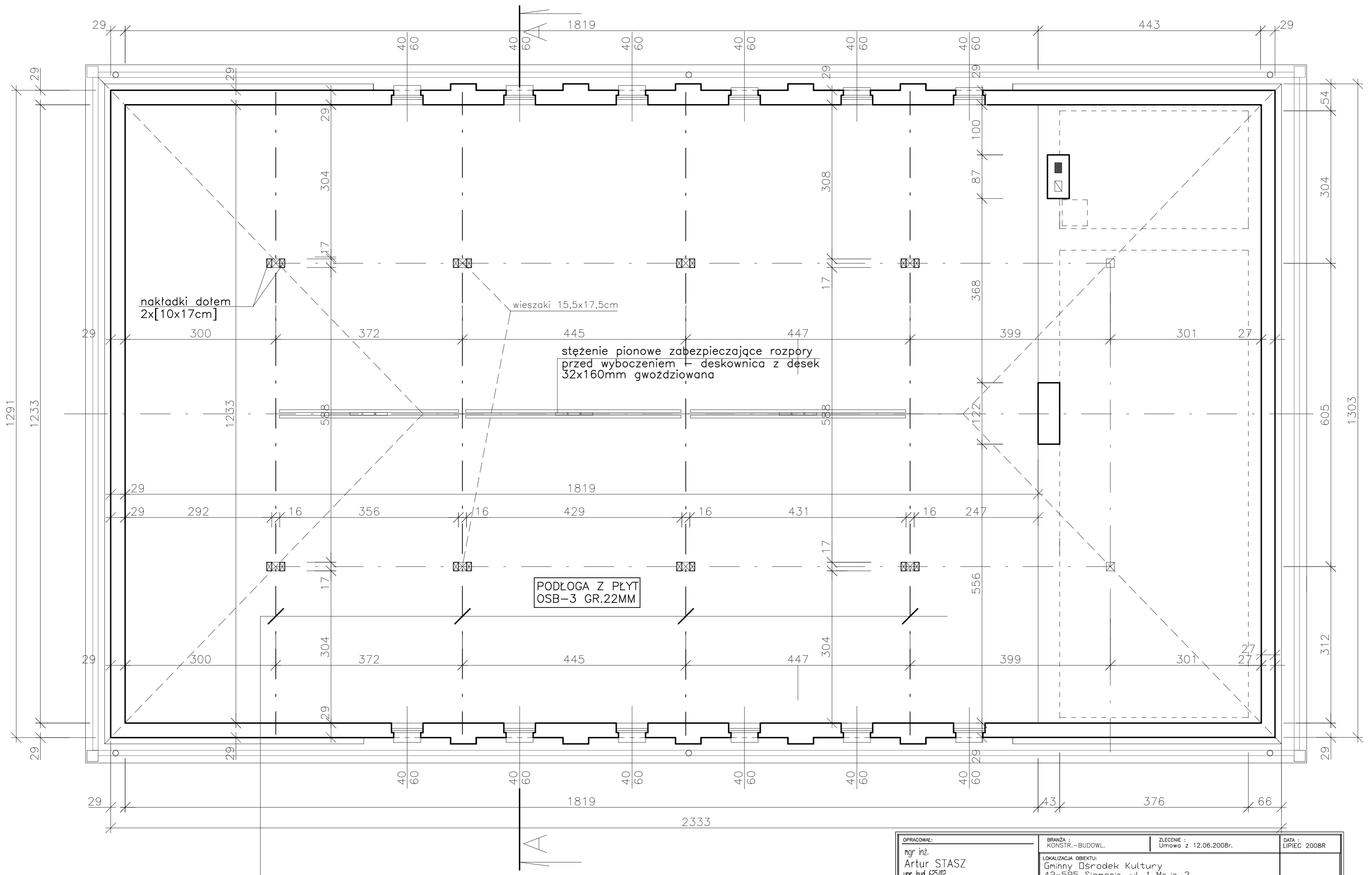
RZUT PODDASZA – 1:50
